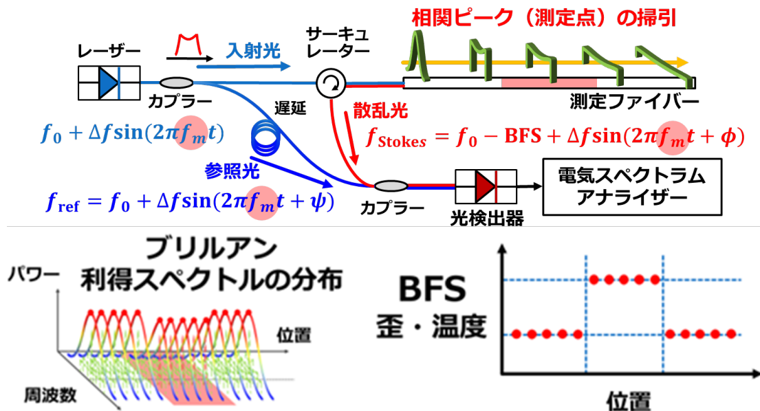
図1. Brillouin光相関領域反射計 (BOCDR) による分布測定の実理：光ファイバーに入射したレーザー光から生じるブリルアン散乱を利用し、ファイバー中の特定の位置だけを選択して温度やひずみを測定する。レーザー光の周波数を制御することで、測定位置をファイバーに沿って移動させ、分布情報を取得することができる。
