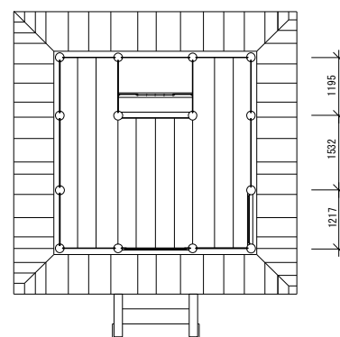
実測調査によるCAD図面(蓮華峰寺弘法堂)
